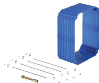
38 896 000 Prodlužovací sada, 50 mm pro 37 338 000 a 38 787 000
